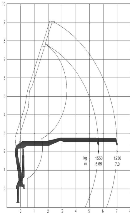
STROMBELASTUNGSPLAN
