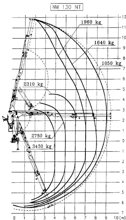
ZÁŤAŽOVÝ DIAGRAM
