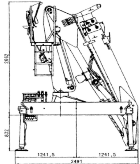
ROZMERY
