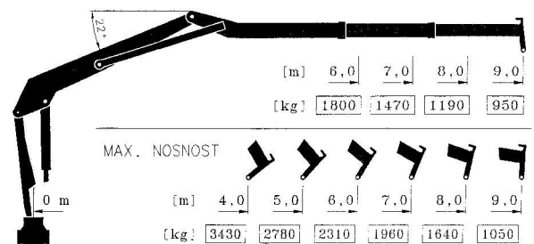
TRAGKRAFTTABELLE
